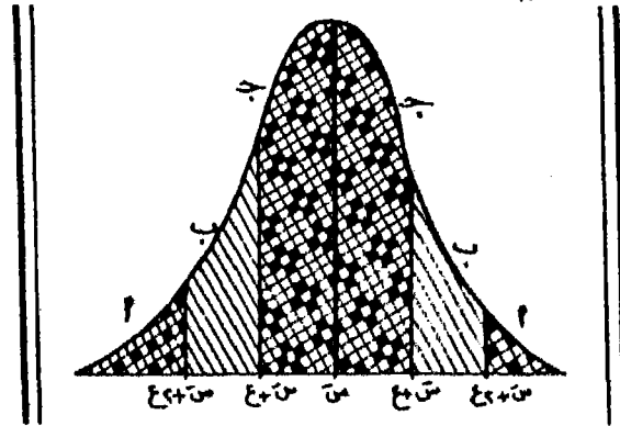
المساحة الواقعة تحت الأجزاء المختلفة من المنحنى الطبيعي
